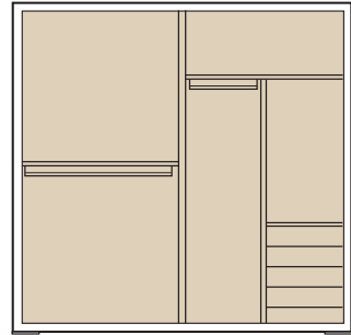
DOTAZIONE INTERNA ARMADIO - 2 ripiani grandi - 1 bastone grande - 1 bastone piccolo - cassetтира interna a 5 cassetti
